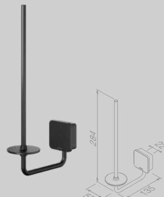
Reserverolhouder Spare toilet roll holder
