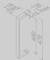
Douchedeurgreep 45 cm Shower door handle 45 cm 913559-02-45
