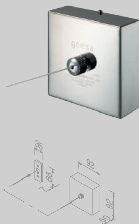
Waslijn uittrekbaar Washing line retractable
