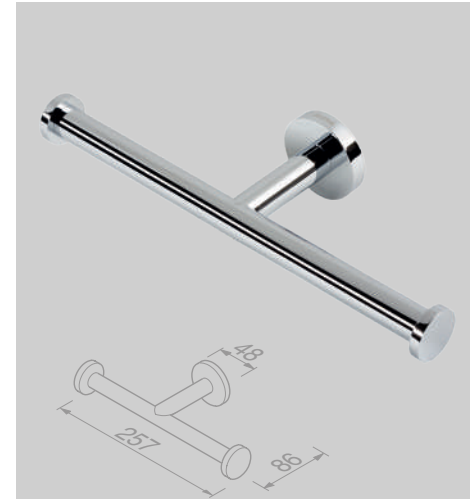
Toiletrolhouder dubbel Toilet roll holder double 916518-02
