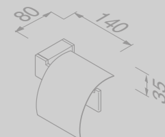
Toiletrolhouder met klep Toilet roll holder with cover
