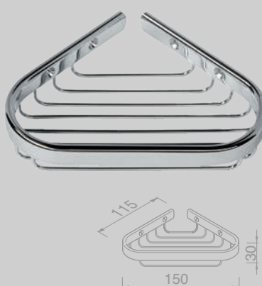
Zeephouder Soap holder 91137A
