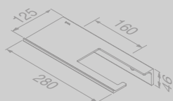
Planchet 28 cm met toilethouder zonder klep Bathroom shelf 28 cm with toilet roll holder without cover
