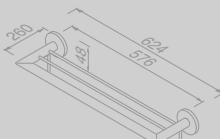
Handdoekrek met planchet 60 cm Towel rail with shelf 60 cm
