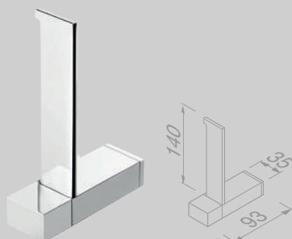
Reserverolhouder Spare toilet roll holder
