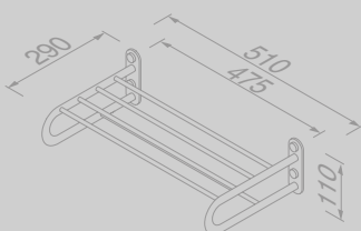
Handdoekrek met planket 50 cm Towel rail with shelf 50 cm 915252
