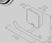
Handdoekhaak dubbel Towel hook double
