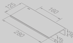
Planchet 28 cm met toilethouder zonder klep dubbel Bathroom shelf 28 cm with toilet roll holder without cover double
