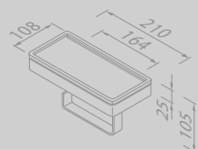
Toiletrolhouder met planket Toilet roll holder with shelf
