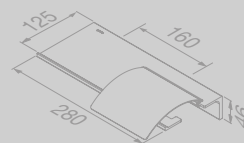
Planchet 28 cm met toilethouder met klep Bathroom shelf 28 cm with toilet roll holder with cover
