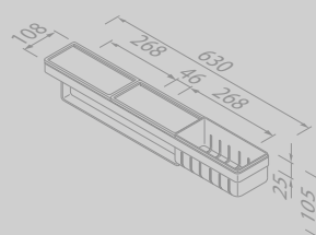
Planket met handdoekrek en douchemand 63 cm Shelf with towel rail and shower basket 63 cm
