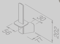
Reserverolhouder Spare toilet roll holder
